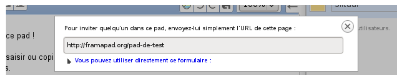
Illustration 8: Fenêtre d'invitation
